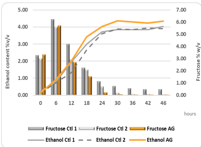
Figure 1: Cinétique de fermentation et concentration en fructose au cours de la fermentation sur jus d'agave. Sélection de DistilaMax AG Mexico 2023
